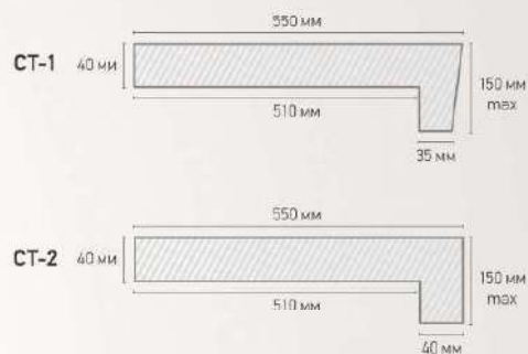
Ступени Г-образные 1200 (max) / 550 (max) / 150 (max) / 40 мм
