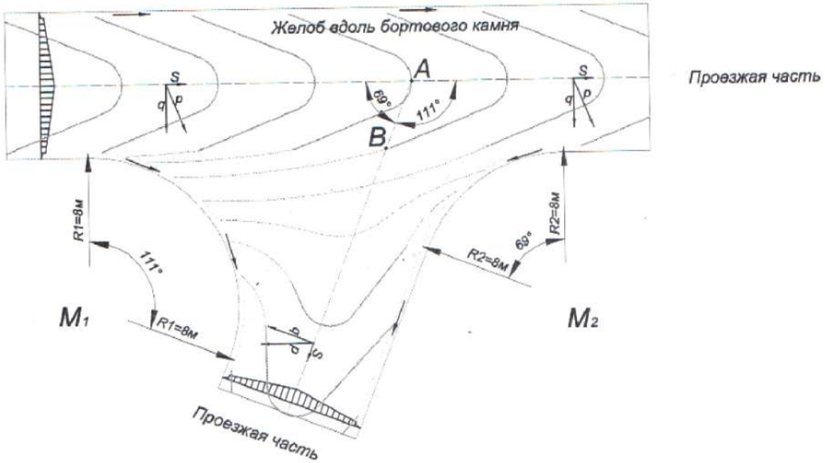
Схема примыкания под углом
