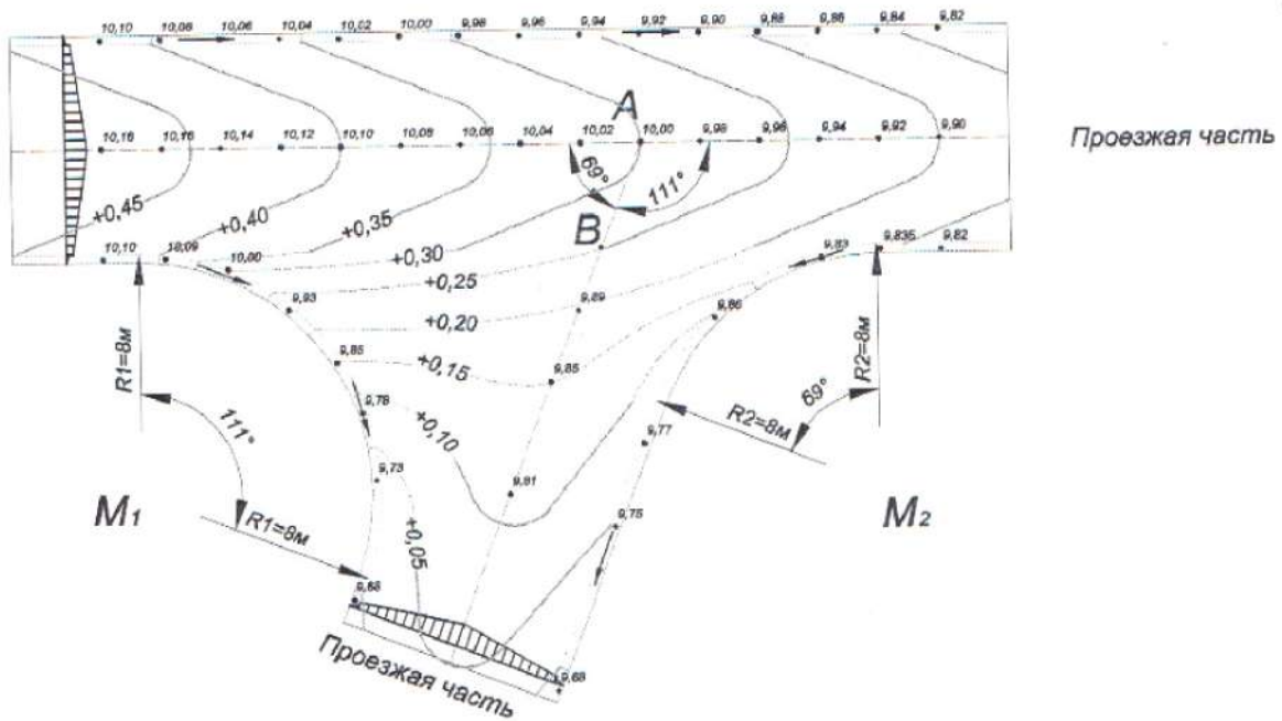
Пример примыкания под углом с высотными отметками
